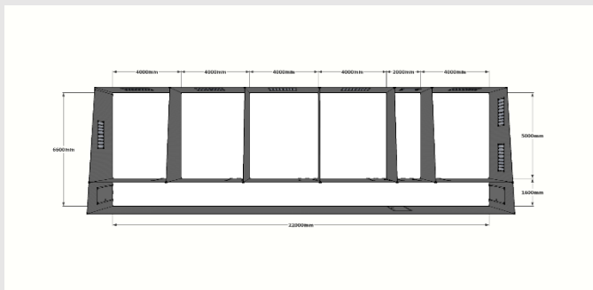
Plan de coupe du bâtiment
